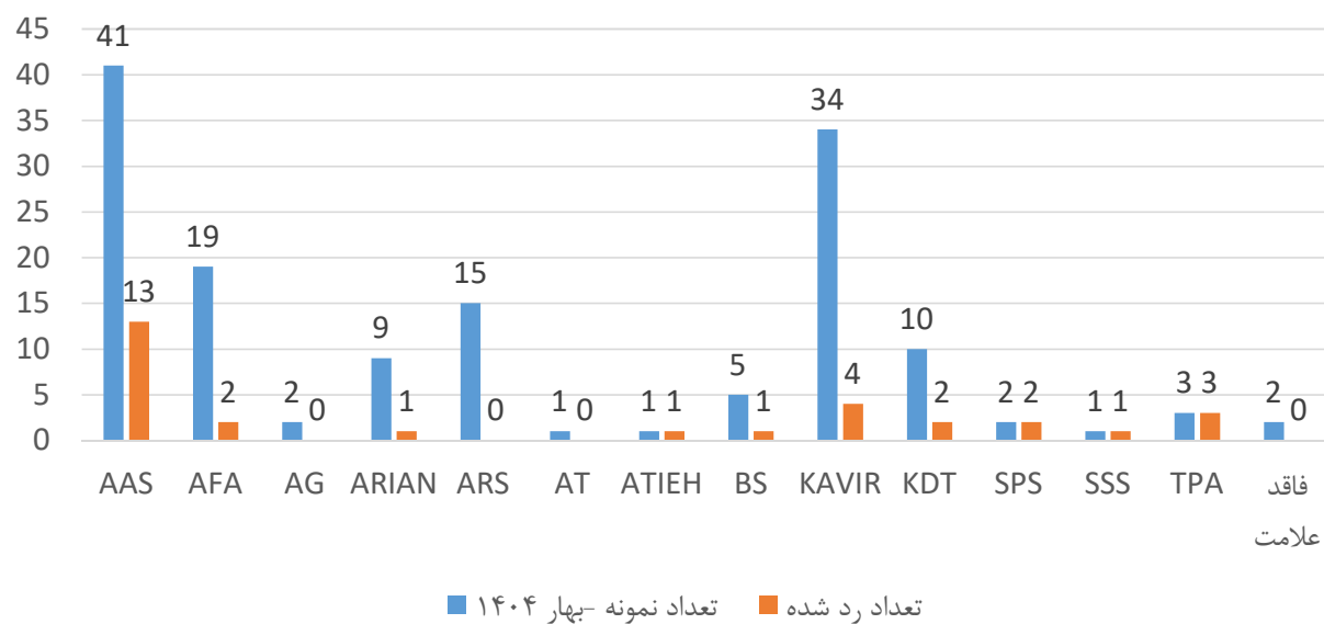
توزیع آماری نتایج در میلگرد T10 در بهار ۱۴۰۴
