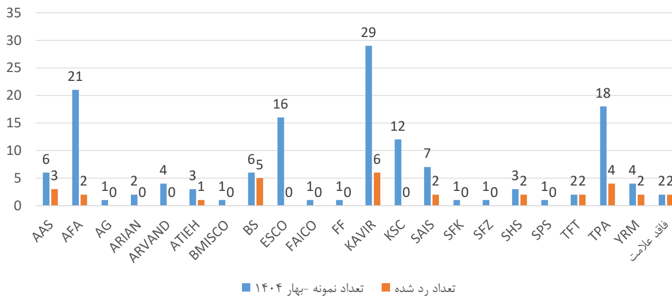
توزیع آماری نتایج در میلگرد T16 در بهار ۱۴۰۴
