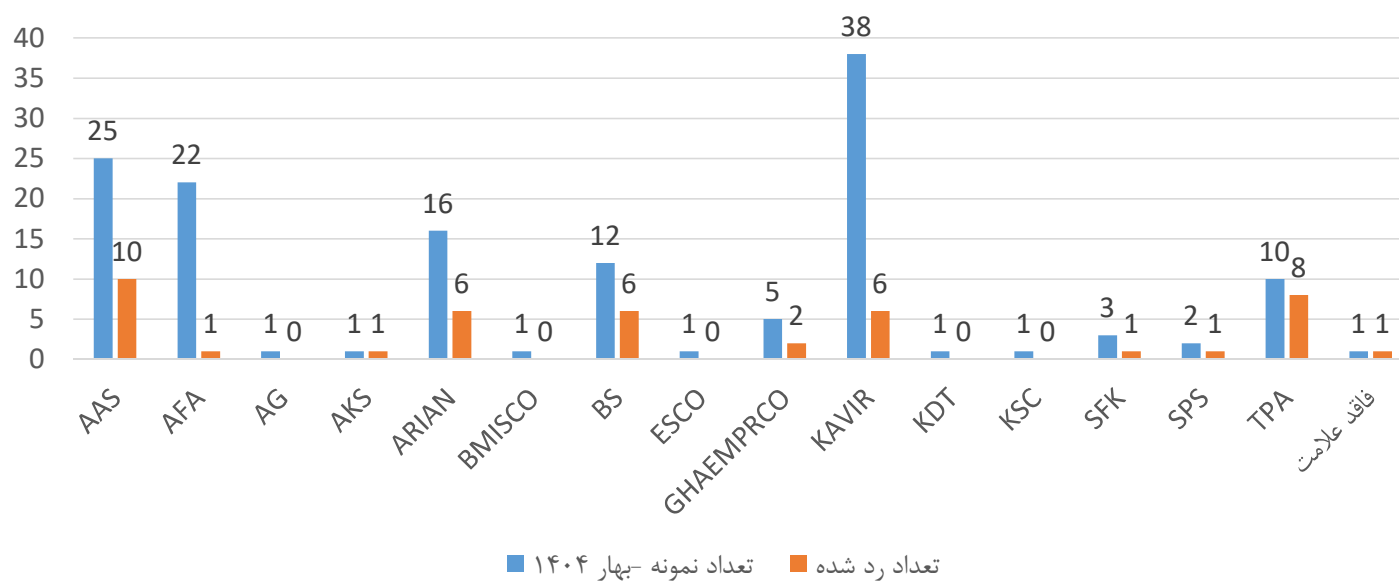
توزیع آماری نتایج در میلگرد T12 در بهار ۱۴۰۴
