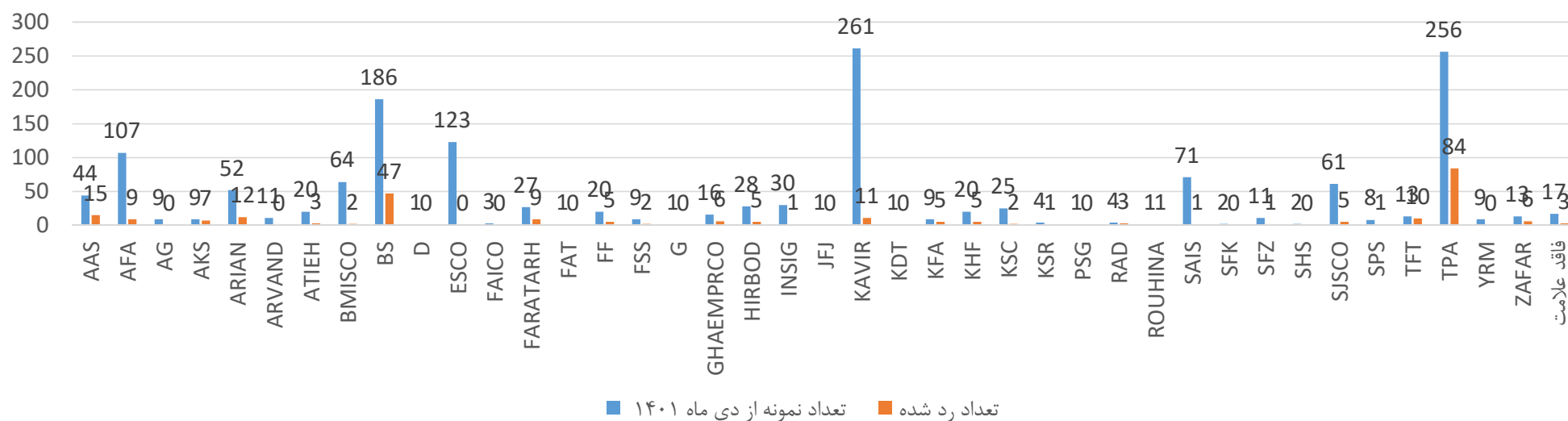
توزیع آماری نتایج در میلگرد T25 از دی ۱۴۰۱ تا خرداد ۱۴۰۴
