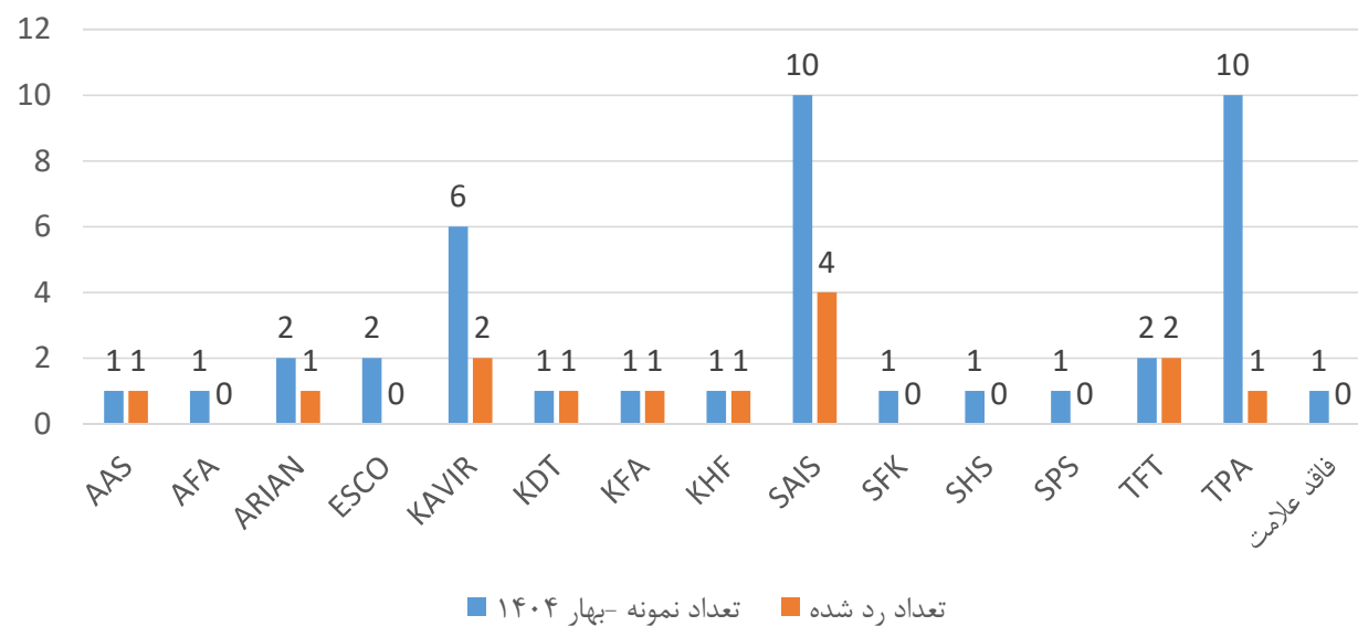
توزیع آماری نتایج در میلگرد T14 در بهار ۱۴۰۴
