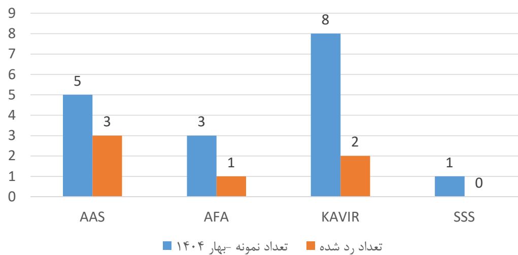
توزیع آماری نتایج در میلگرد T8 در بهار ۱۴۰۴
