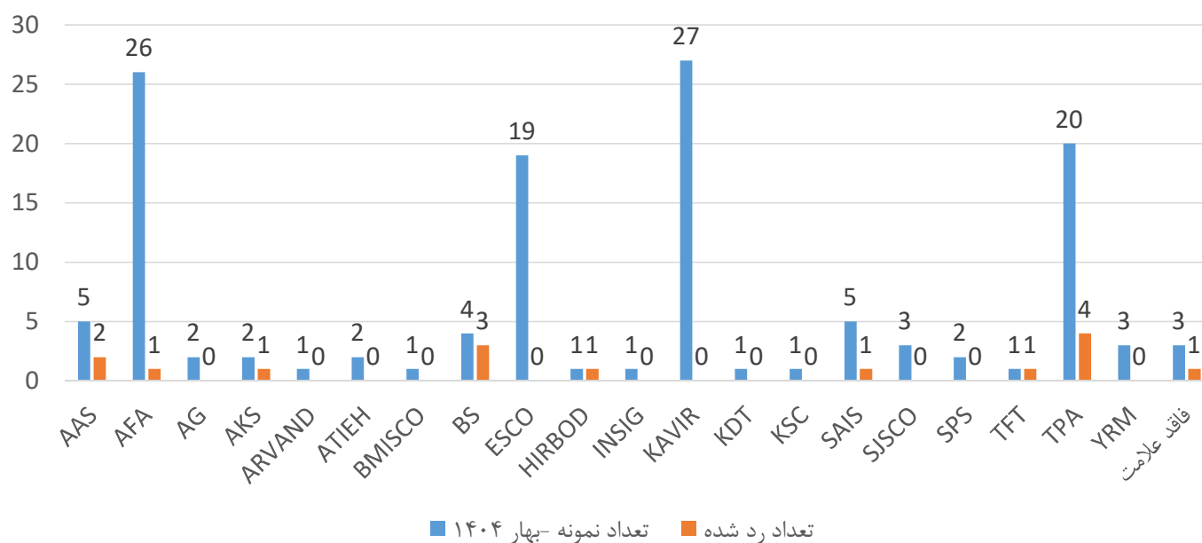
توزیع آماری نتایج در میلگرد T25 در بهار ۱۴۰۴
