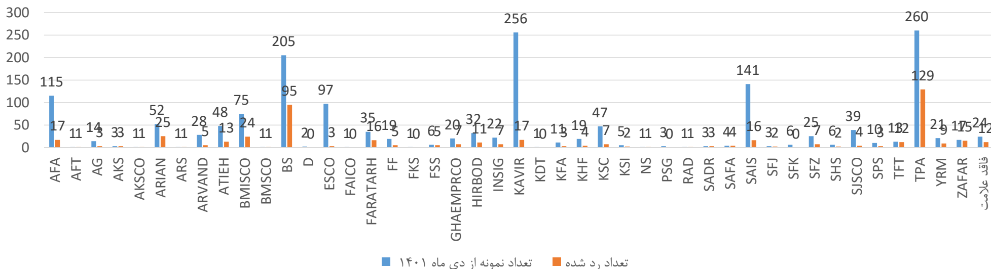
توزیع آماری نتایج در میلگرد T16 از دی ۱۴۰۱ تا خرداد ۱۴۰۴
