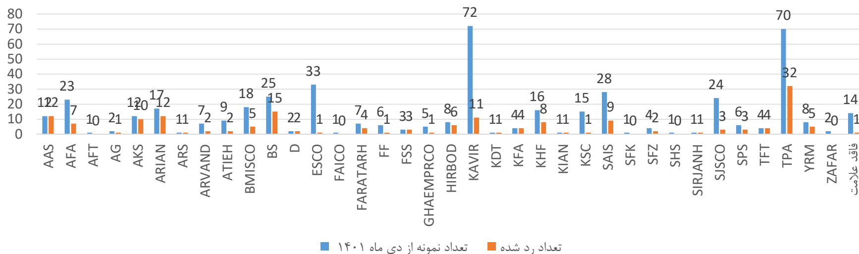
توزیع آماری نتایج در میلگرد T14 از دی ۱۴۰۱ تا خرداد ۱۴۰۴
