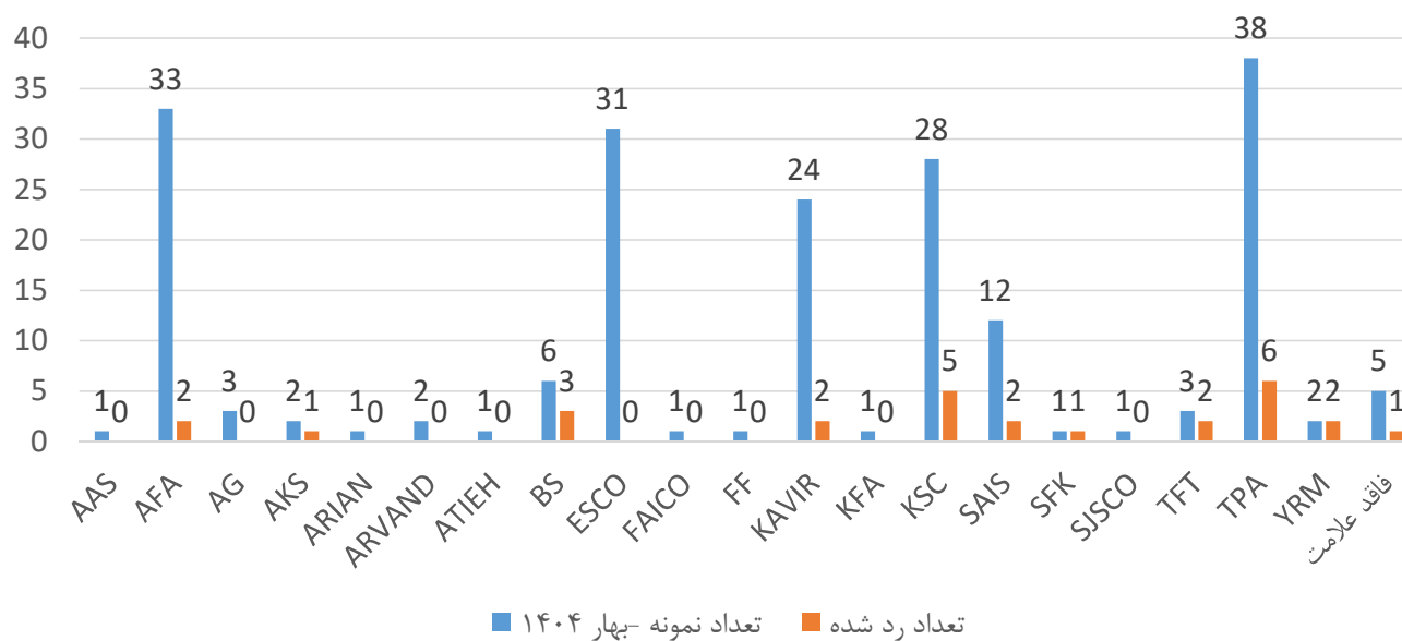
توزیع آماری نتایج در میلگرد T20 در بهار ۱۴۰۴
