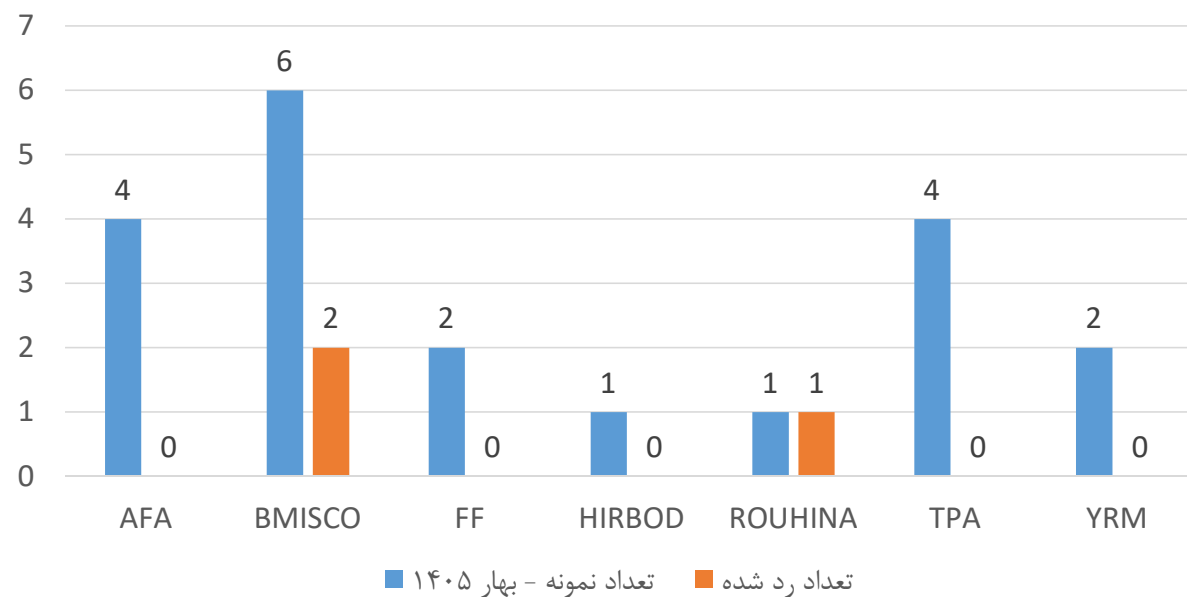
22 توزیع آماری نتایج در میلگرد T در بهار ۱۴۰۵
