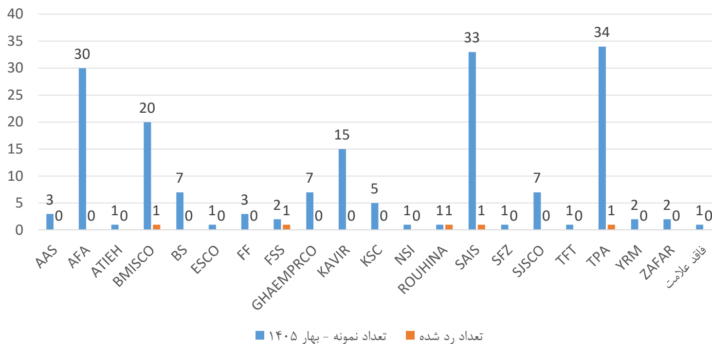
25 توزیع آماری نتایج در میلگرد T در بهار ۱۴۰۵
