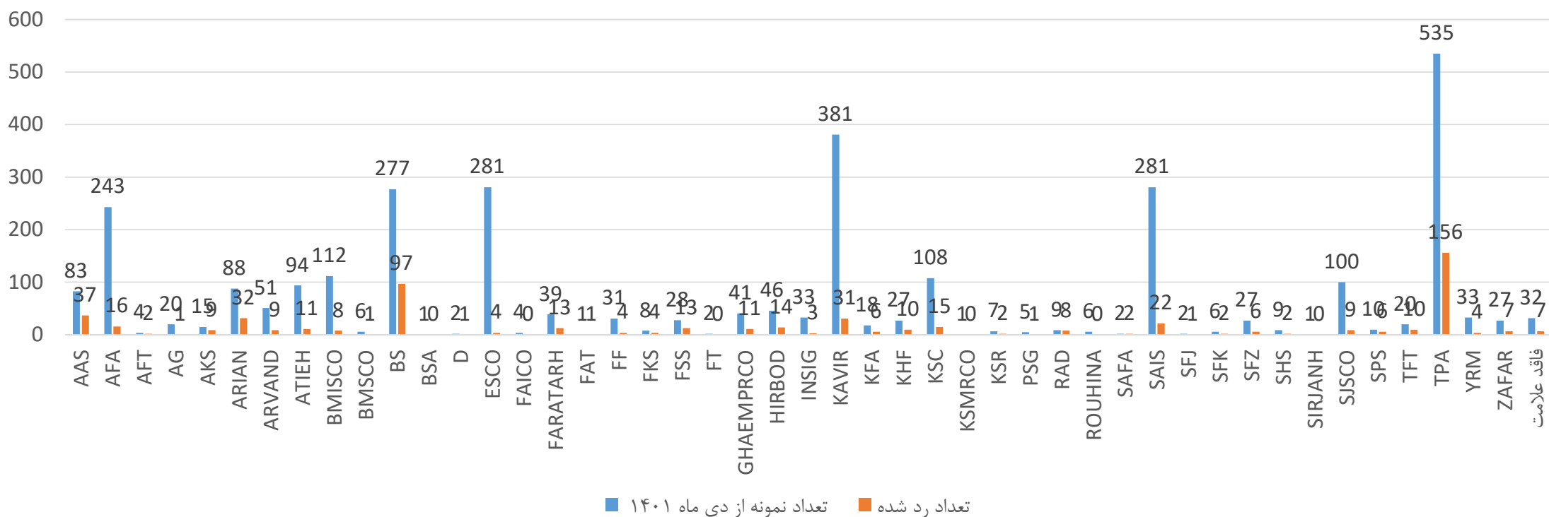
توزیع آماری نتایج در میلگرد T20 از دی ۱۴۰۱ تا خرداد ۱۴۰۵
